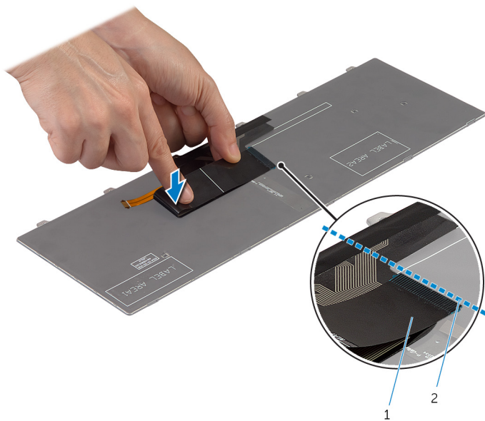
1 billentyűzetkábel
